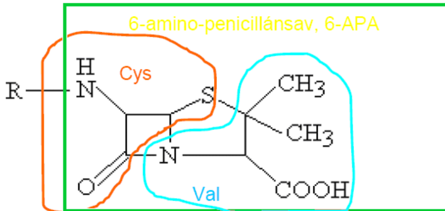
5. ábra: A penicillin molekula felépítése
