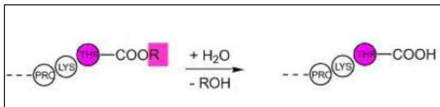
21. ábra: Az észter csoport elbontása
