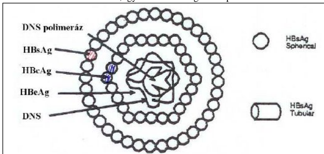
26. ábra: A Hepatitis B vírus felépítése
