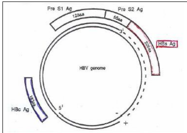
27. ábra: A Hepatitis DNS-e
