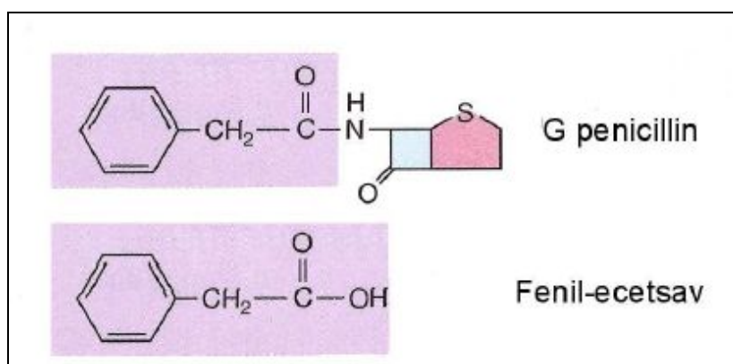
9. ábra: A fenil-ecetsav mint prekursor
