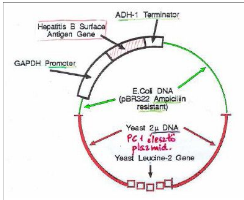
28. ábra: Az élesztőbe bevitt plazmid szerkezete
